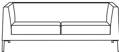
W: 1810 H: 700 D: 810 SH: 430
